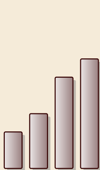
run1
